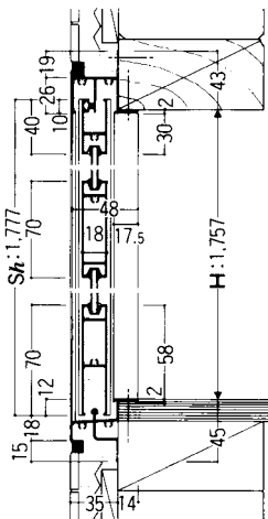
縦断面図 ①-①
