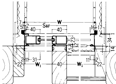
横断面図 ②-②
