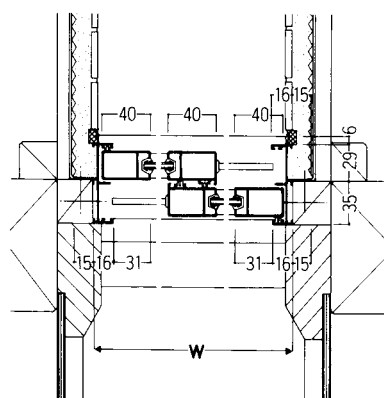
横断面図 ⑥-⑥
