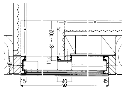
横断面図 ④-④
