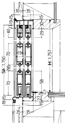
縦断面図 ⑤-⑤
